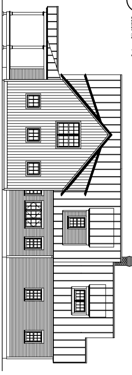
5 SOUTH ELEVATION Scale: 1/8" = 1'-0"
