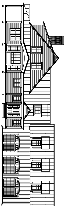
4 WEST ELEVATION Scale: 1/8" = 1'-0"
